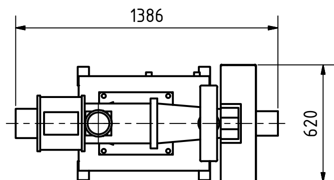
A ( 1 : 20 )
