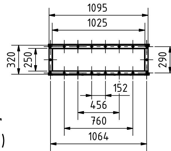
Inlet A ( 1 : 25 )
