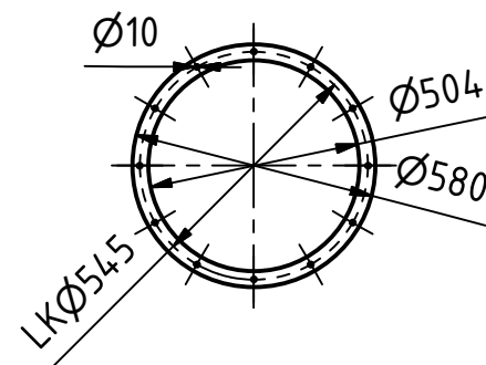
Aspiration ( 1 : 20 )
