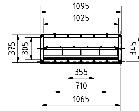
Outlet B ( 1 : 25 )
