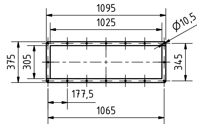
Outlet ( 1 : 20 )
