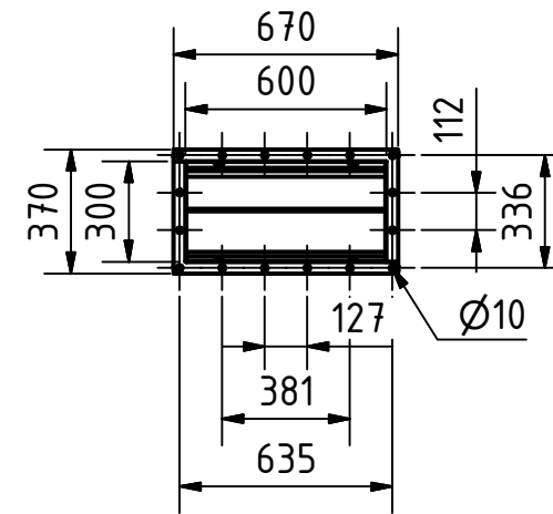
Auslauf B ( 1 : 25 )
