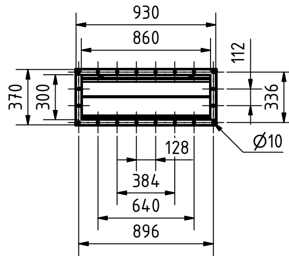
Auslauf B ( 1 : 25 )
