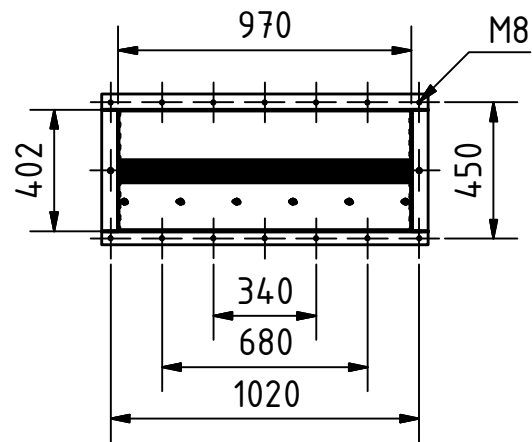
Einlauf A ( 1 : 25 )
