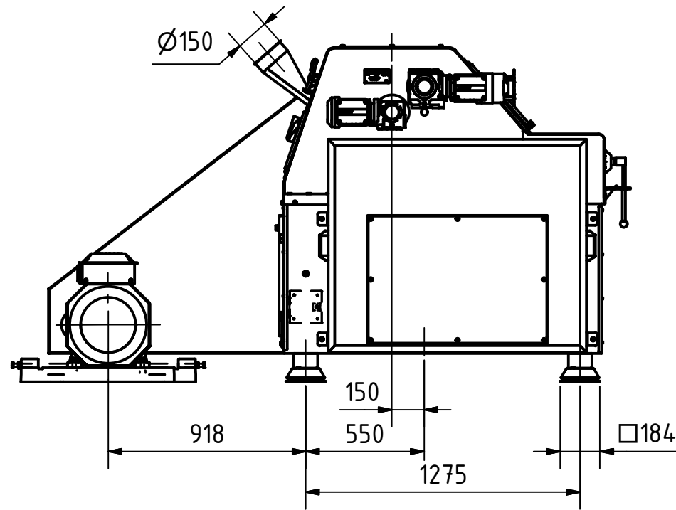
Einlauf A ( 1 : 25 )
